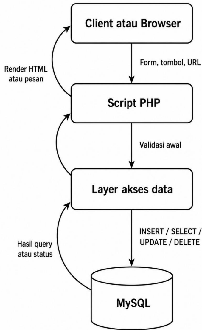
Gambar 2.1 Flowchart implementasi dasar PHP CURD dalam pengembangan web
